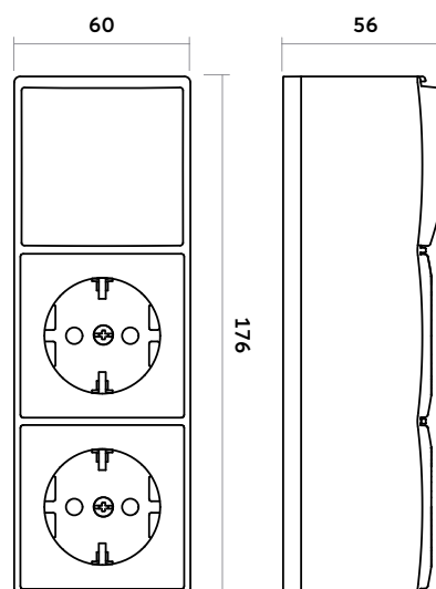
Kombination Doppelsteckdose mit Wippschalter
