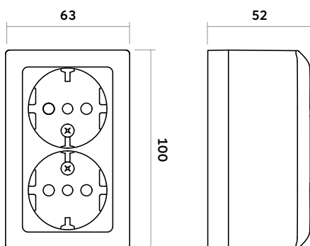
Steckdose 2-fach
