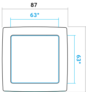
Schalter
