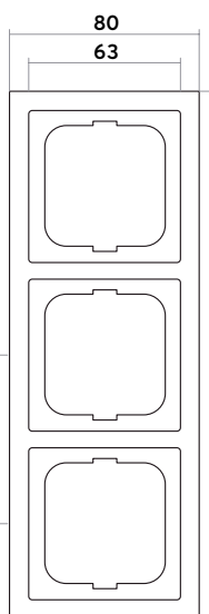
Abdeckrahmen 3-fach
