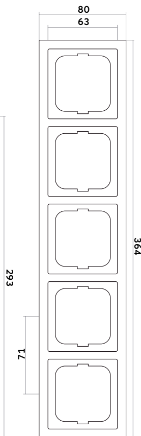
Abdeckrahmen 5-fach
