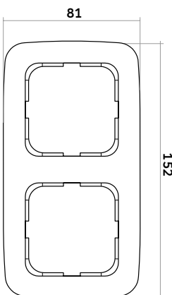
Abdeckrahmen 2-fach
