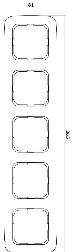
Abdeckrahmen 5-fach
