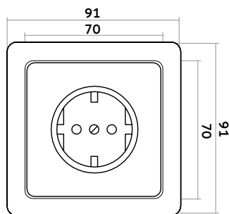
Steckdose
