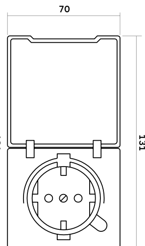
SCHUKO® Steckdosen-Einsatz mit Klappdeckel
