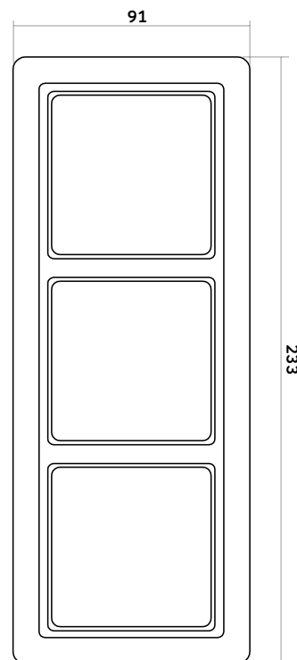
Abdeckrahmen 3-fach
