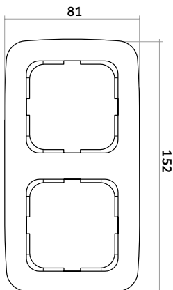
Abdeckrahmen 2-fach
