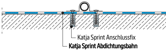
F4504.de-V5 Rohrschelle auf Rohboden
