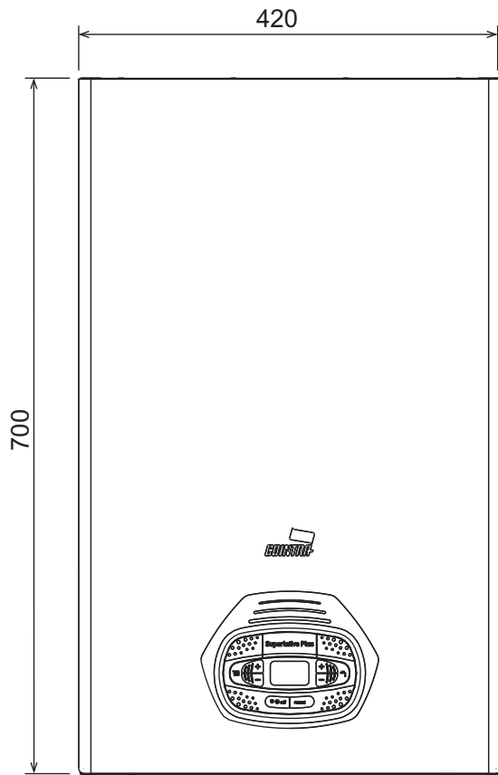
fig. 52 - Vista frontal
