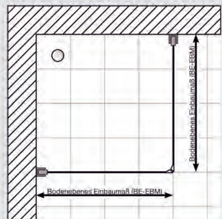
Montage Bodeneben
