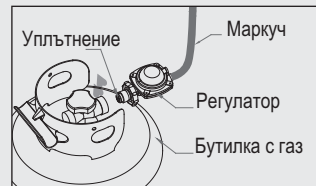
Свързване на маркуча с регулатора и на регулатора с газовата бутилка
