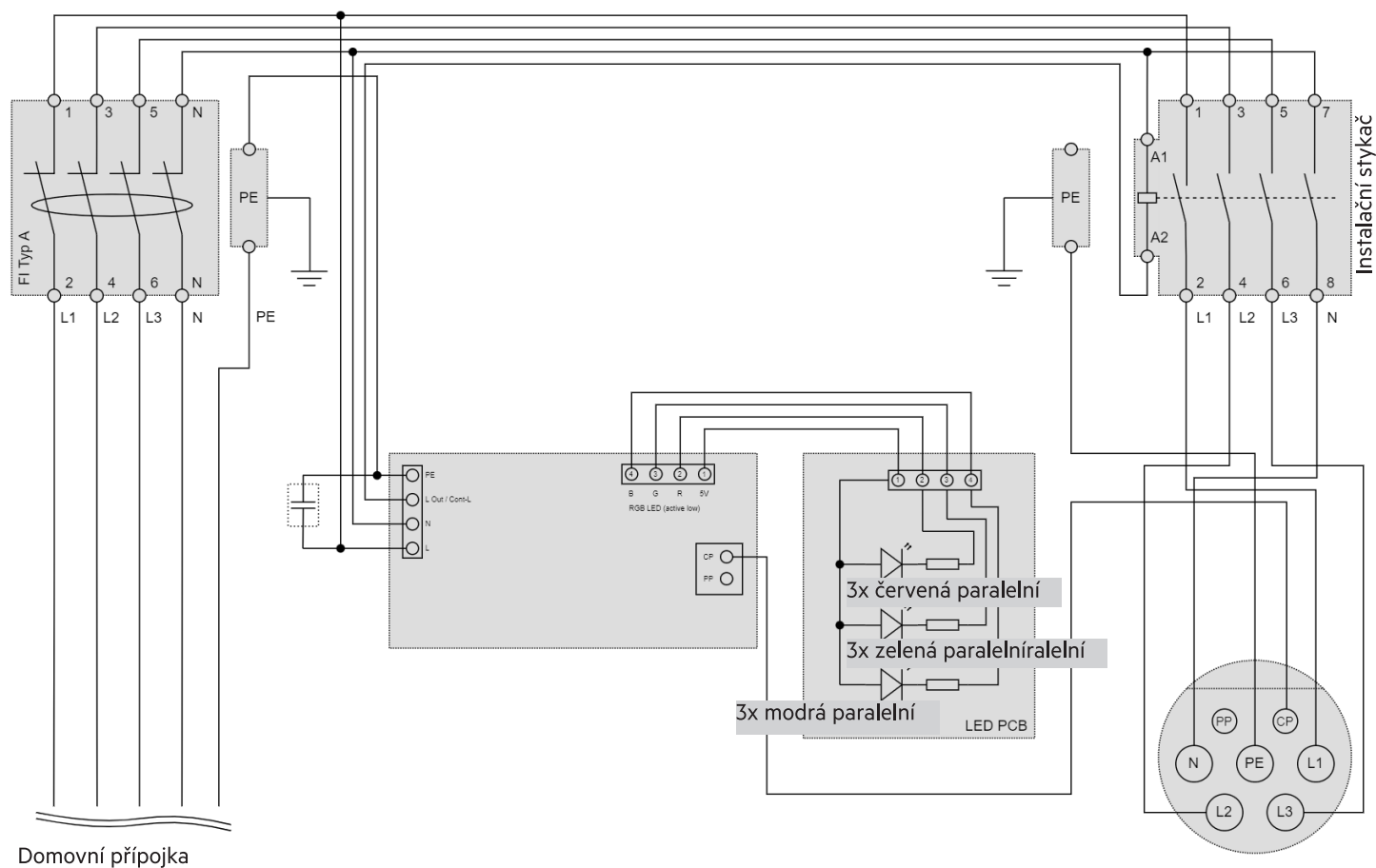
Obr. 4: Schéma zapojení AEG Wallbox Pro
