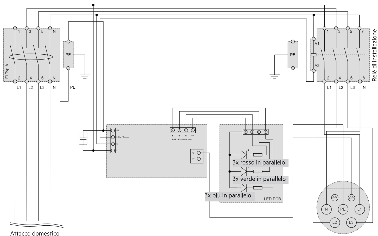
Fig. 4: Schema elettrico AEG Wallbox Pro
