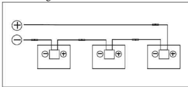
String-Verbindung
