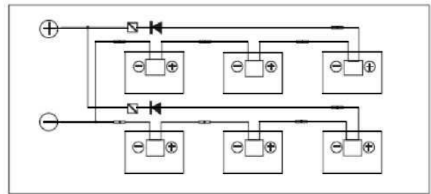
Parallele Verbindung
