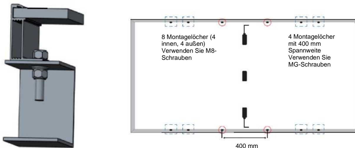
Abbildung 6 Schematische Darstellung 1 des monofacialen Moduls mit Schraube, Installation
