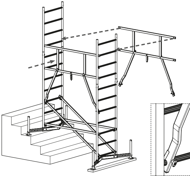
2 x Art.-No. 710673
