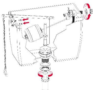
Dibujo técnico
