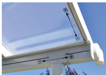
Podesivi položaj stupova
