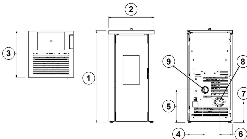
Fig. 12 - Allgemeine Abmessungen: VERA 7 - VERA 7.0
