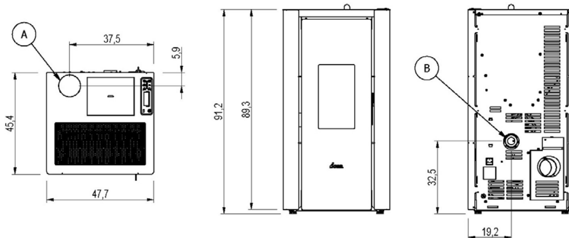
Fig. 15 - Allgemeine Abmessungen: CRISTAL3 7.0 UP
