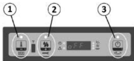
Fig. 24 - 3-Tasten-Display
