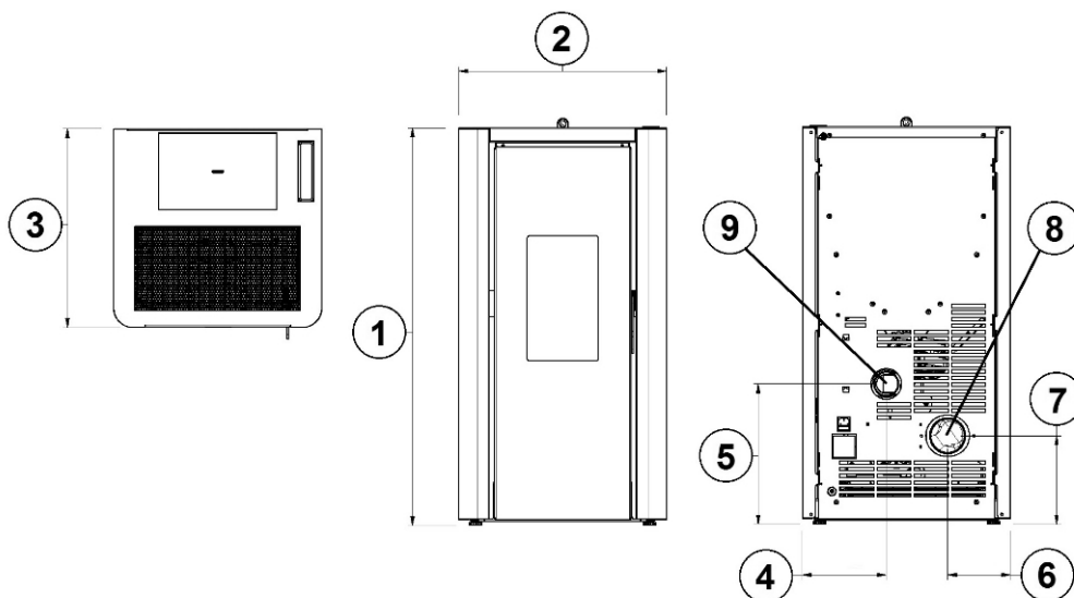
Fig. 13 - Allgemeine Abmessungen: INDIGO EVO - INDIGO EVO 7
