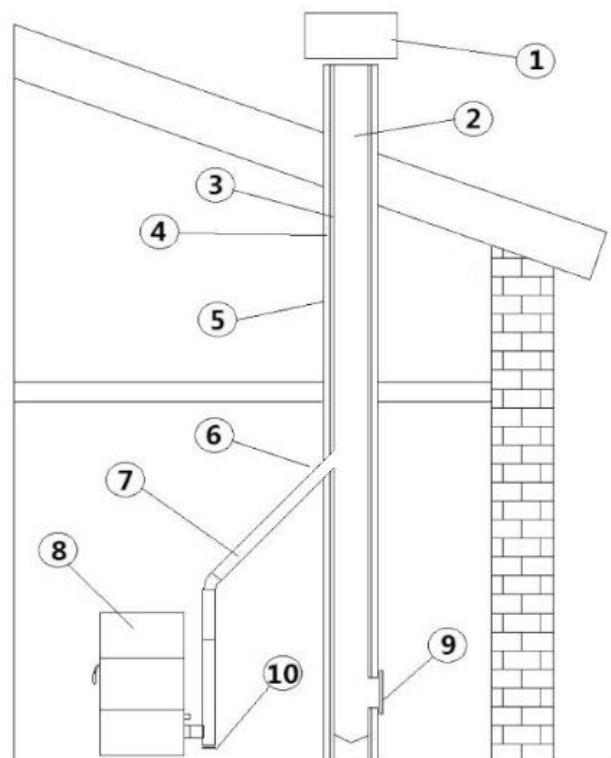
Fig. 2 - Bauteile Kamin
