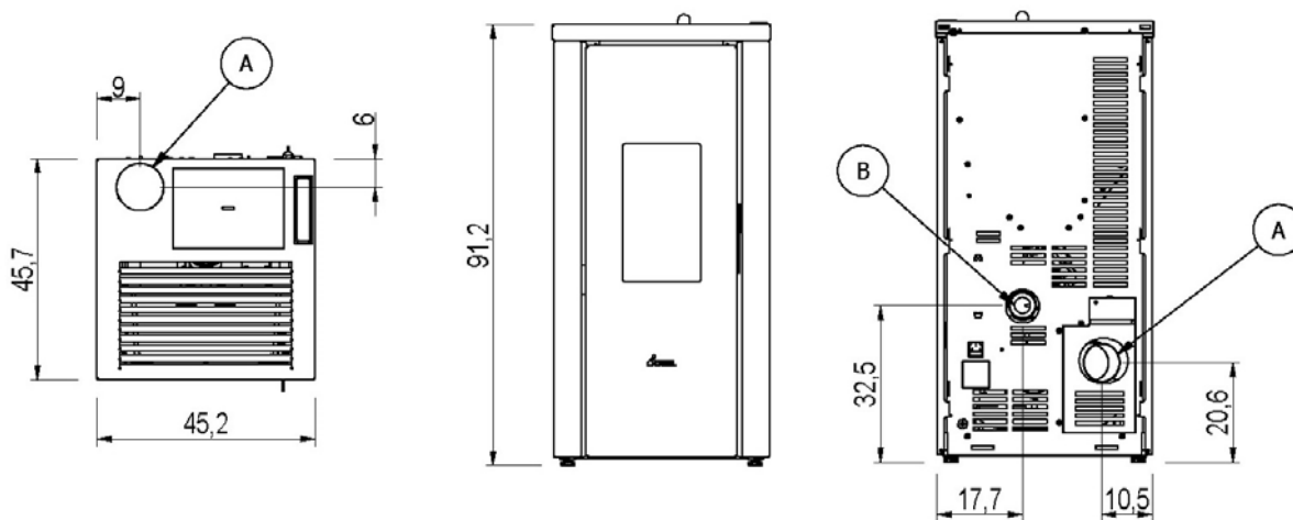
Fig. 14 - Allgemeine Abmessungen: VERA 7.0 UP
