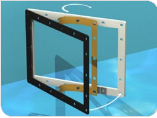
Abbildung 43 – Der zweite Flansch
