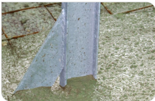
Abbildung 11 – Giessen der Betonplatte (c)
