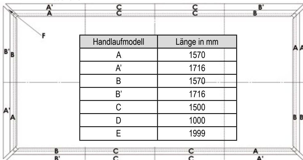
Abbildung 46 – Handläufe - Weva 3 x 6
