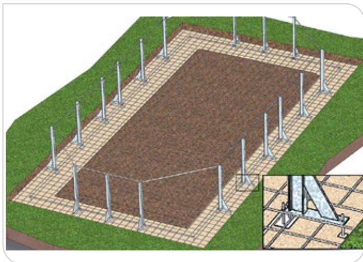
Abbildung 9 – Giessen der Betonplatte (a)
