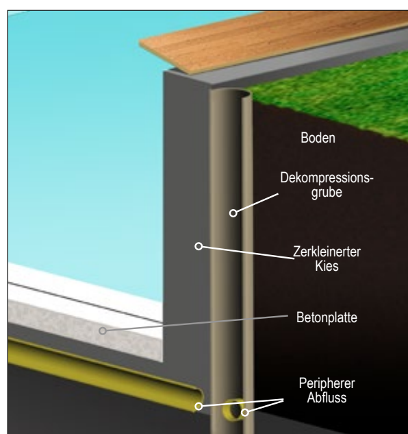
Dränage
