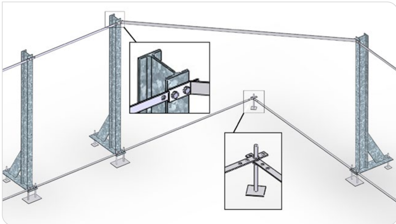
Abbildung 6 – Metallträger
