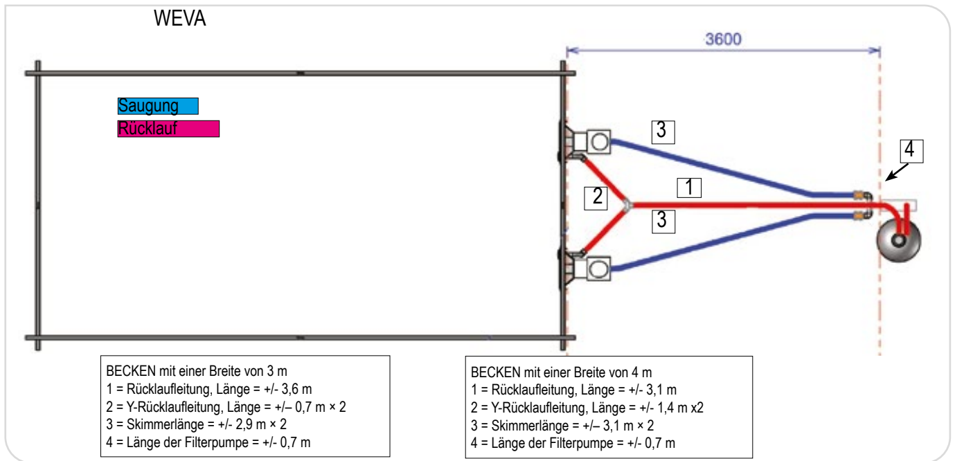
Abbildung 39 – Beispiel für die Filtration mit zwei Skimmern - Weva
