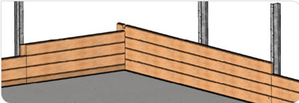
Abbildung 17 – Montage der Wände
