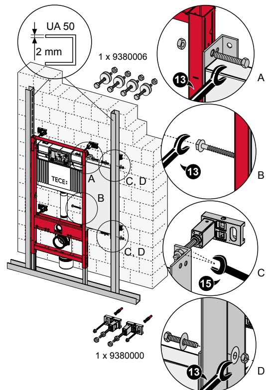
Einbau in eine Metallständerwand
