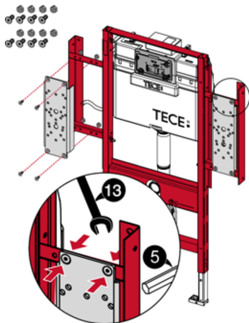
Montage der seitlichen Stahlplatten an das Gerontomodul
