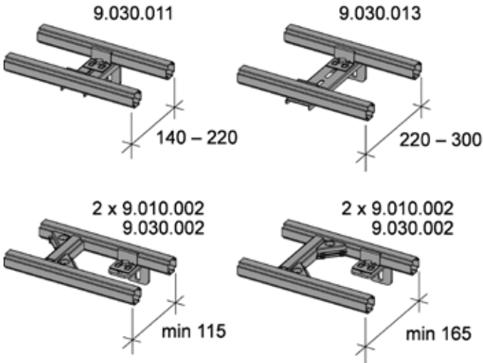
Mögliche Vorwandtiefen mit TECEprofil Tragwerk
