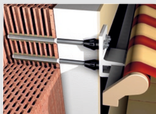
Markisenbefestigung
