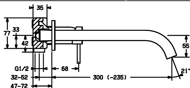
Produktzeichnung
