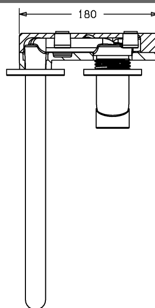
Produktzeichnung
