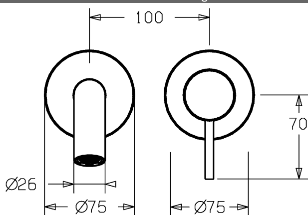
Produktzeichnung
