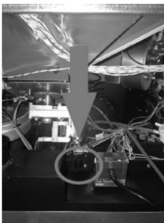
Fig. 42 - Rearme manual: está ubicado detrás del depósito, cerca de la toma de alimentación.
