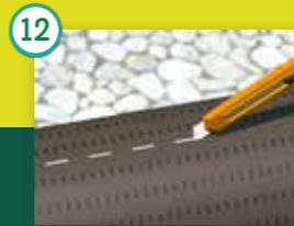
12 Ajustar las piezas entre sí, retirar el sobrante con un cúter
