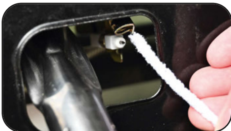
Pilottipolttimen puhdistus hetulalangalla tai piipunpuhdistimella.
