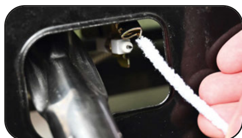
Limpiar el quemador piloto con un alambre de chenilla o un limpiapipas.
