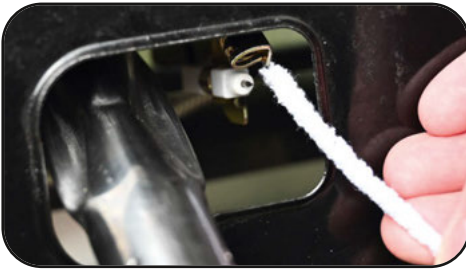
Pilot yakıcının bir lif teli veya bir pipo yardımı ile temizlenmesi.
