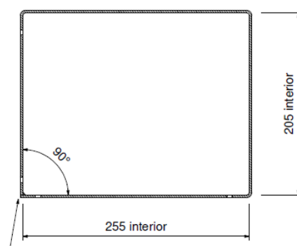
sección A-A'
