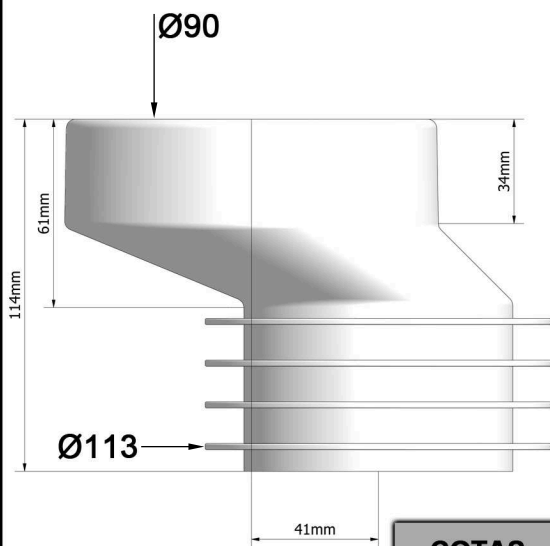
COTAS
