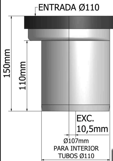
COTAS
