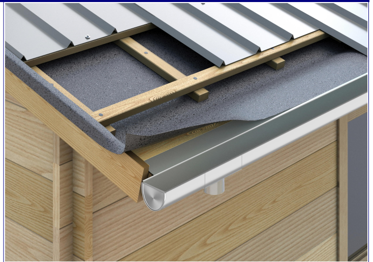
Anwendungsbild
