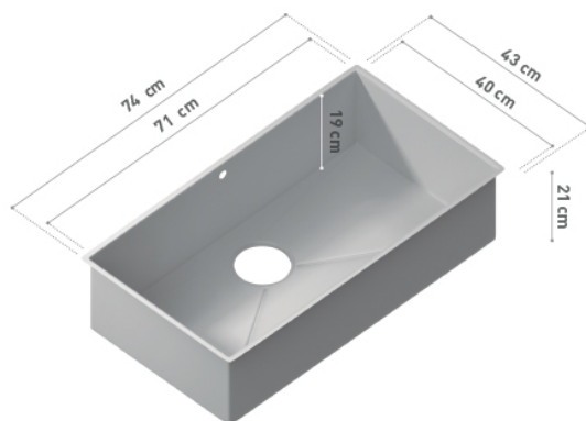
DIBUJO 2 AXONOMÉTRICO
