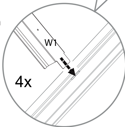
Cadre de base de l'abri de jardin floraworld à toit 2 pans I
