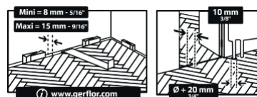
DEHNUNGSFUGENABSTAND
