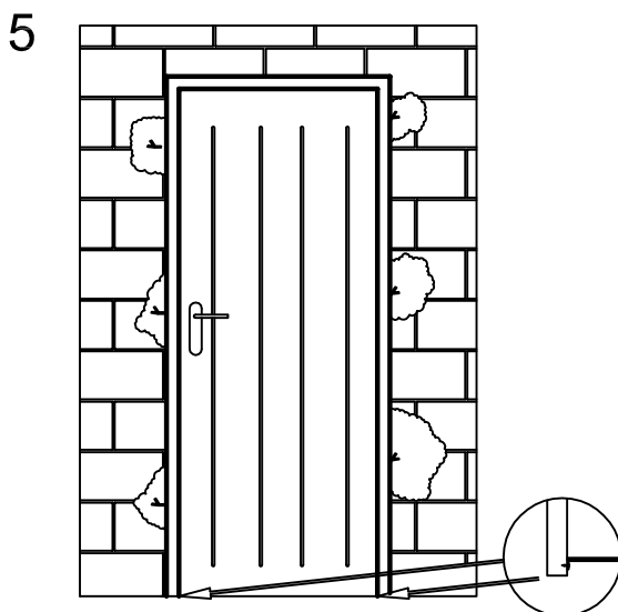
5. Una vez se este seguro de que el mortero está completamente seco, abra la cerradura, accione la manilla, y abra la puerta. Se desprenderán los 3 rectángulos de plástico, situado en los burlones de las cerraduras y que ha mantenido las holguras perfectas entre la hoja y el marco, durante su colocación. Posteriormente debe de quitar la riostra de la parte inferior.
