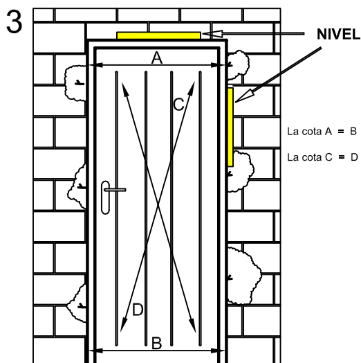
3. Colocar a nivel y comprobar holguras
