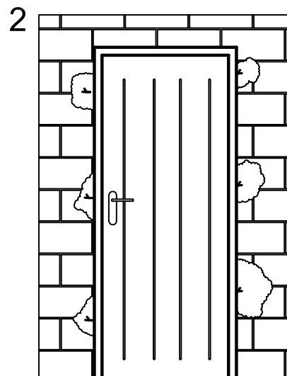
2. Una vez posicionada la puerta, debemos de Abrir las garras, marcarlas y abrir los huecos correspondientes
