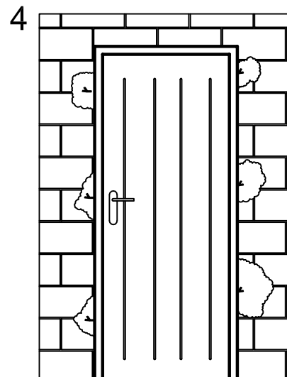
4. Prefijar la puerta con las garras con mortero o similar. Fijar en primer lugar la pata de la bisagra. Volver a comprobar las holguras y nivel. En caso de no ser correcta soltar la fijación y comenzar de nuevo.
