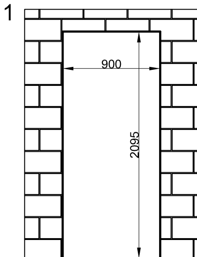
1. Comprobar medida del hueco
