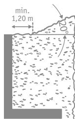
C | Böschung Geländeneigung 30^\circ (bis 155 cm Höhe) / 5^\circ (ab 180 cm Höhe) (105 cm Höhe ausgenommen)
