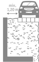
E | Verkehrs- last bis p = 5 \text{ kN/m}^2 , mit Ver- dichtungsdruck e_{vh} = 25 \text{ kN/m}^2 , Abstand: 1,2 m (bis 155 cm Höhe)/ 1,5 m (ab 180 cm Höhe) (55-105 cm Höhe ausgenommen)
