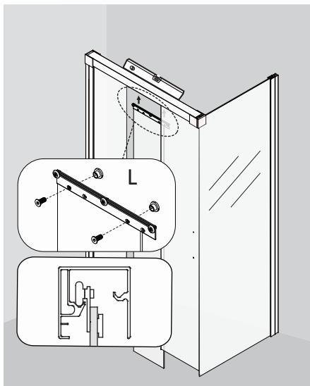
8A Colocar guía superior a corredera central y colgarla en perfil superior
