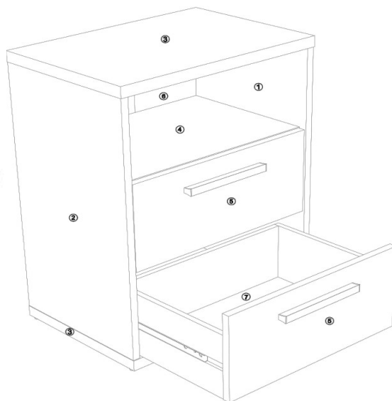
⑥ Trasera 610x231x3 Painel Traseiro - Back Panel - Panneau D'Arrière
