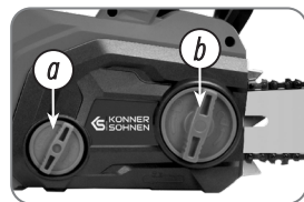
a). Kettenzugmutter b). Abdeckungsdruckmutter
