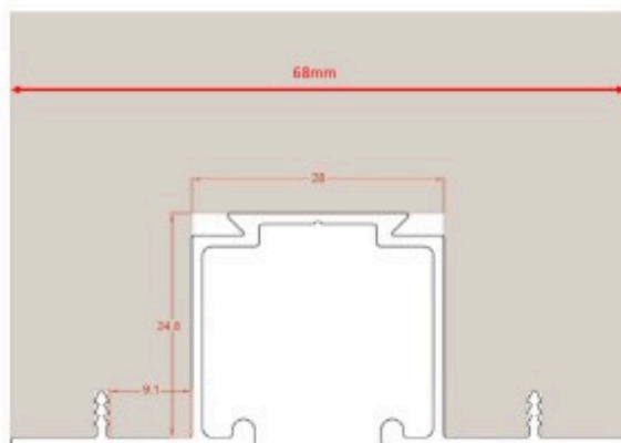
Dibujo con cotas del producto
