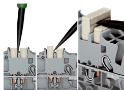
Kammbrücke lösen Mit dem Betätigungswerkzeug zwischen Brücke und Trennsteg der Brückenschächte eintauchen und Brücke heraushebeln. Bei Brücken (5-fach) Betätigungswerkzeug mittig ansetzen (siehe Abb. 3), ab 5-fach wechselseitig.
