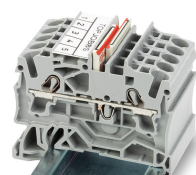
Schachtelbrücke mit dem roten Streifen innenliegend anordnen. Den Schachtelbrücke einsetzen und bis zum Anschlag hinunterdrücken.
