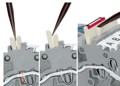
Schachtelbrücke lösen. Um den Schachtelbrücke zu lösen, mit dem Betätigungswerkzeug zwischen den Brücken eintauchen und den Brücke heraushebeln.
