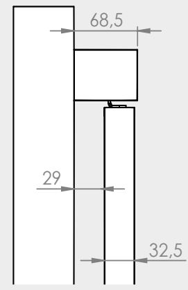
mit Abstandsprofil With spacer profile
