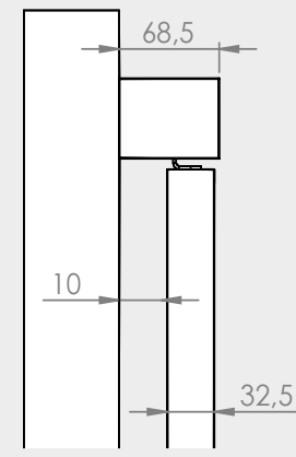
ohne Abstandsprofil Without spacer profile
