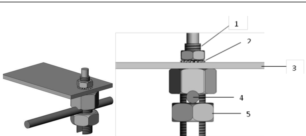
Abbildung 4. Tyco-Erdungsbolzen Nr. 2058729-1
