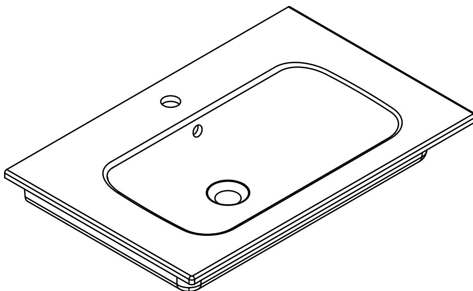
Keramikbecken 710x15x465 mm weiß Ceramic basin 710x15x465 mm white
