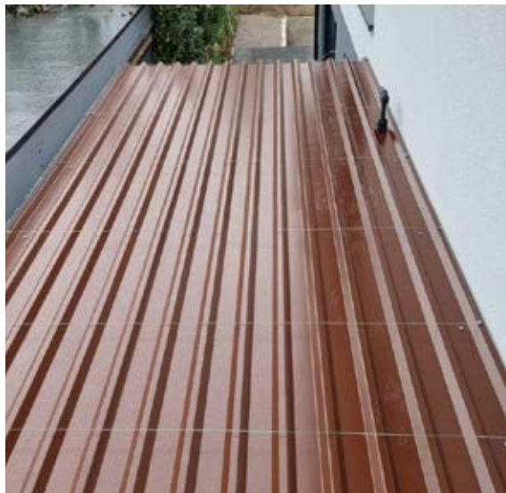
Schnur über jede Pfette spannen
