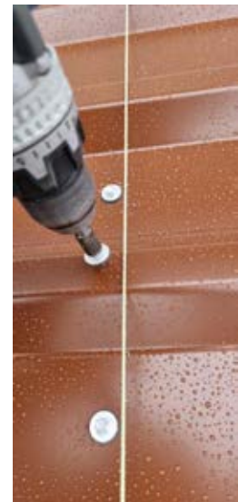
An der Schnur entlang das Dach mit den Pfetten verschrauben
