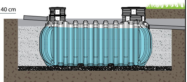
Montage der UNGROUND EXTENSION – Aufsätzen unter schwierigen Bedingungen mit einheimischem Boden und Entlastungsschicht.
