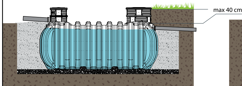
Montage der UNGROUND EXTENSION mit einheimischem Boden
