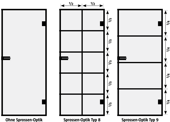
Türhöhe 1972 mm
