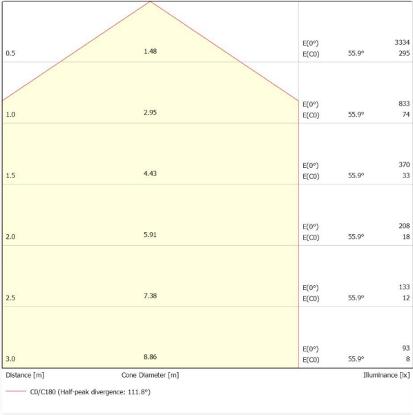
Diagrama de cono DLM20SGW
