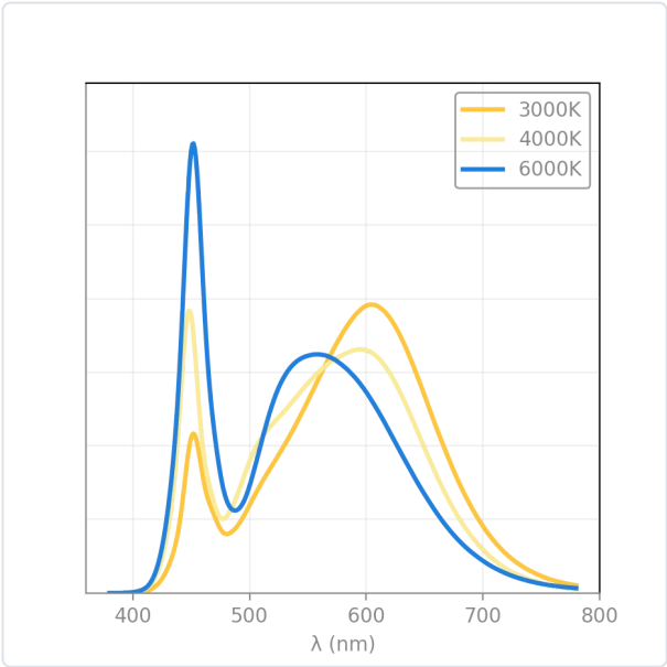
Distribución espectral DLM20SGW
