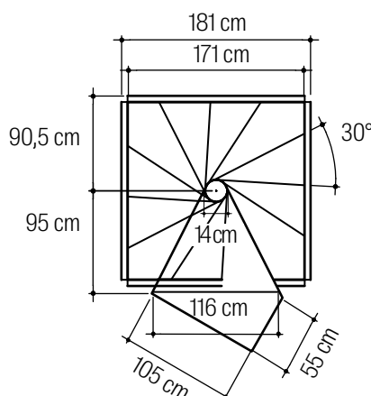
Diámetro 180 cm
