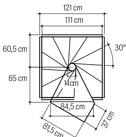
Diámetro 120 cm
