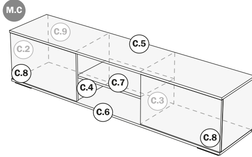
C.1 Costado Derecho 368x380x16 Lateral Derecho - Right Side - Côté Droit
