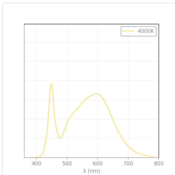
Distribución espectral P5DLE054B
