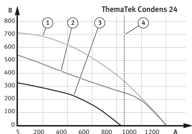
Curvas de la bomba de calefacción (muestran la relación entre presión y caudal)
