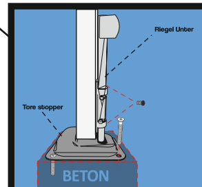
MONTAGE DER TORVERRIEGELUNG
