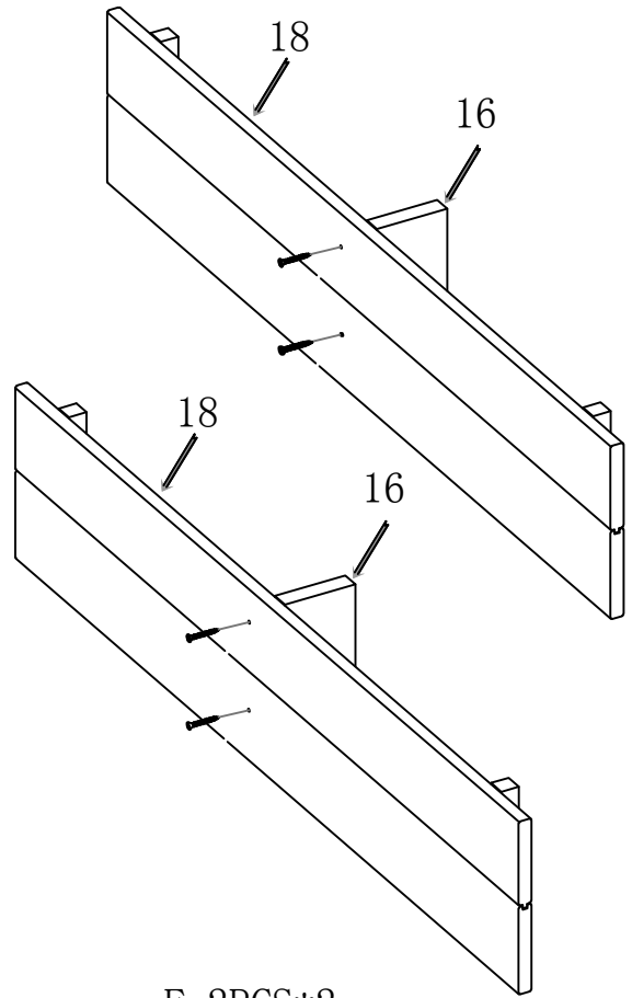
F 2PCS*2
