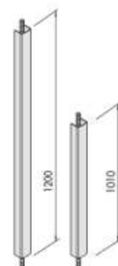
Varillas roscadas y perfil de protección para cierre superior e inferior de la hoja pasiva
